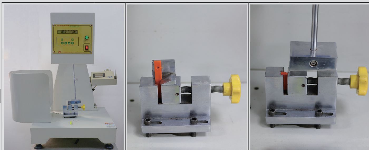
Machine d'essai Charpy
